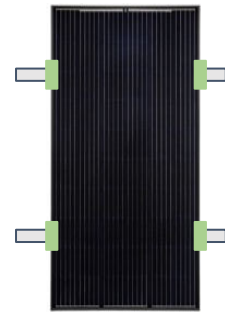
Platzierung der Modulklemmen
